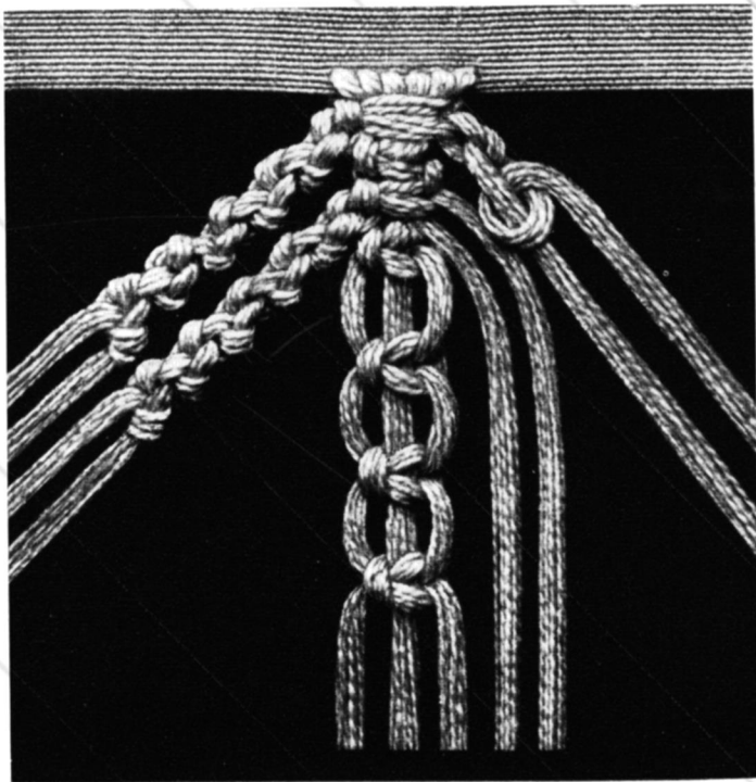
Fig. 15. Manière d'exécuter les chaînettes à nœuds de feston.
